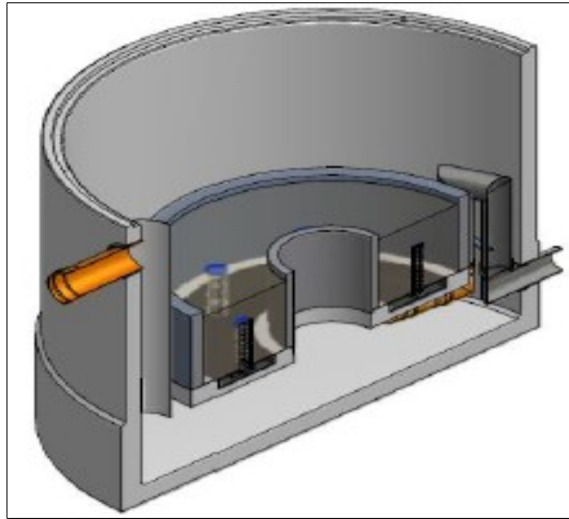
Spaccato esemplificativo dell'impianto
